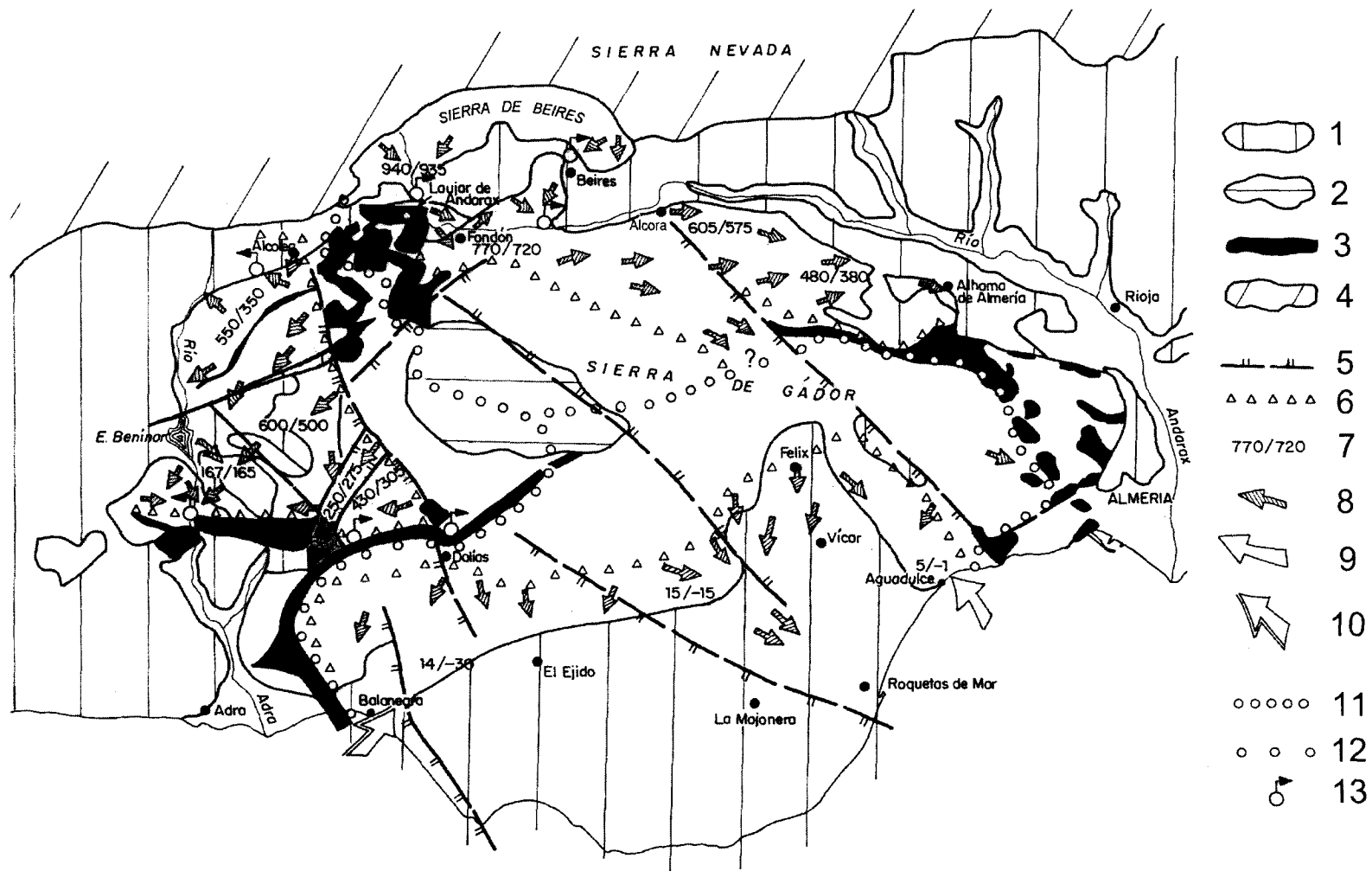
Figura 1: Esquema de funcionamiento hidrogeológico general del sistema de Sierra de Gádor (acuíferos principales). Leyenda: 1=coberteras alpujarrides y/o neógenas del tramo acuífero principal, en conjunto prácticamente impermeables; 2=área aprox. con filitas basales de la U. de Gádor a unos 1000±100 msnm; 3=permotriásico de la U. de Gádor aflorante a subaflorante; 4=impermeable del C. Nevado-Filábride; 5=falla normal con relevancia hidrogeológica; 6=límite de área de acumulación; 7=niveles piezométricos históricos; 8=sentido resultante del flujo subterráneo principal (zona saturada); 9 y 10=entrada de agua marina, directa al AIN y por la cobertera al AIO, respectivamente; 11=divisoria hidrogeológica aproximada; 12=zona de posible transferencia de flujos del Alto Anadarax al AIN del Campo de Dalías (base impermeable del M. de Gádor a unos 800-700 msnm); 13= manantial/galería relevante.
